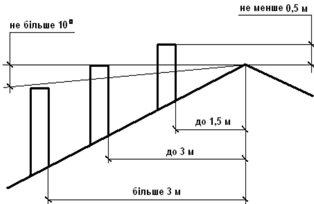
Рисунок 6. Розміщення димоходу
