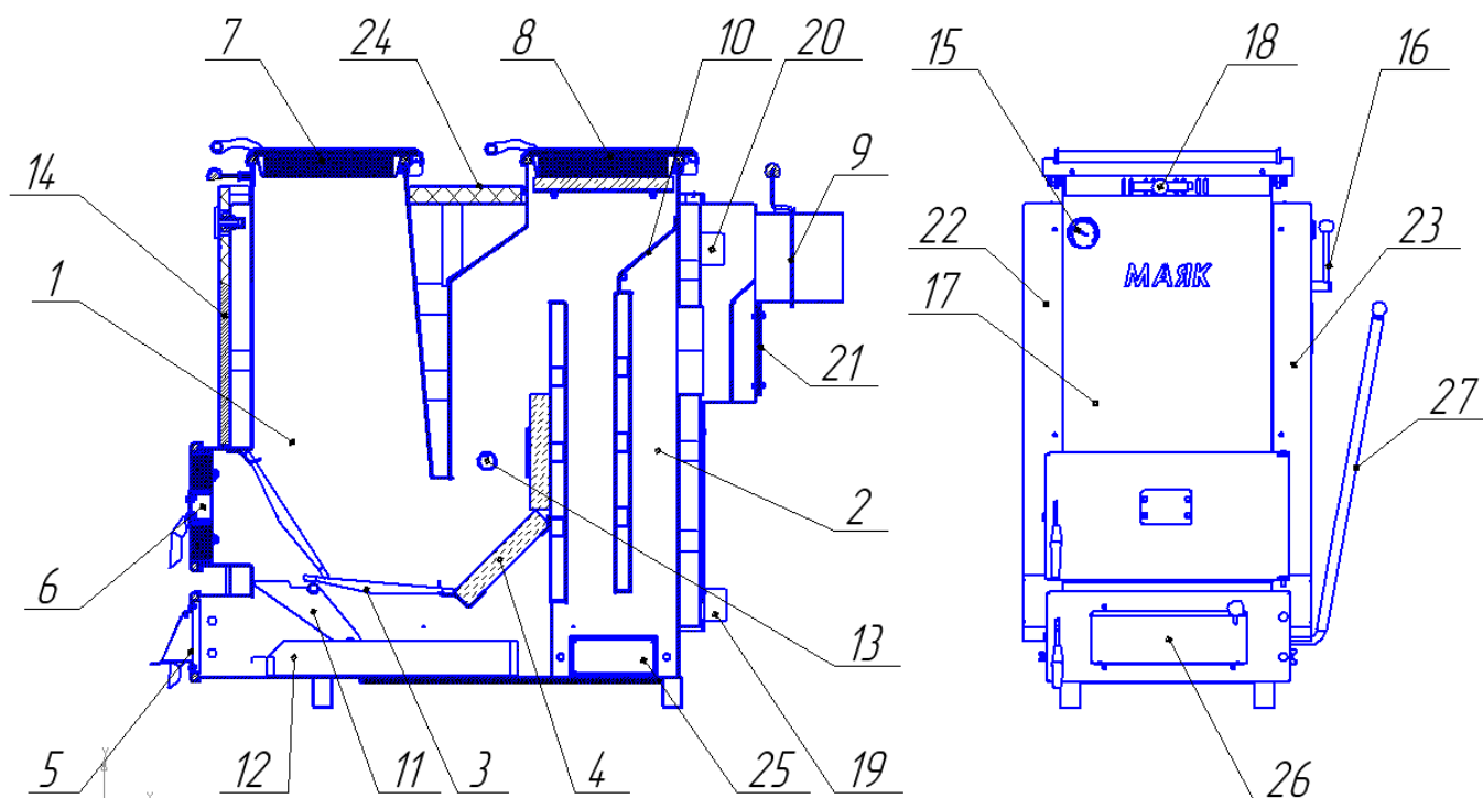
Рисунок 1. Котел опалювальний КТШ ECO LONG BURNING
